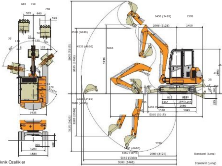
Teknik Özellikler (Kabinli – Kaçuk Palet / Kabinli – Çelik Palet) Standart (Long)
